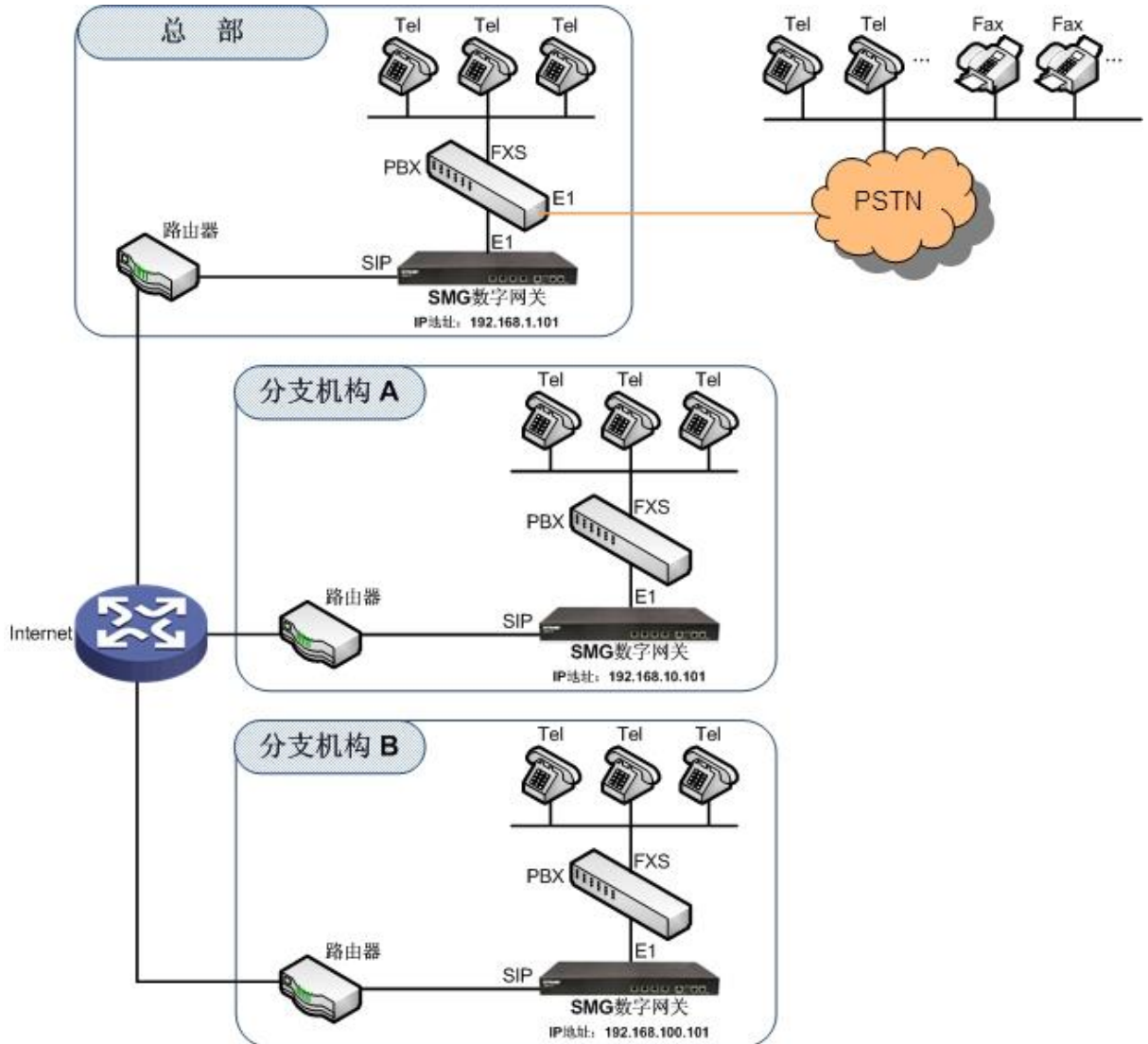
图 4-1 典型应用一
